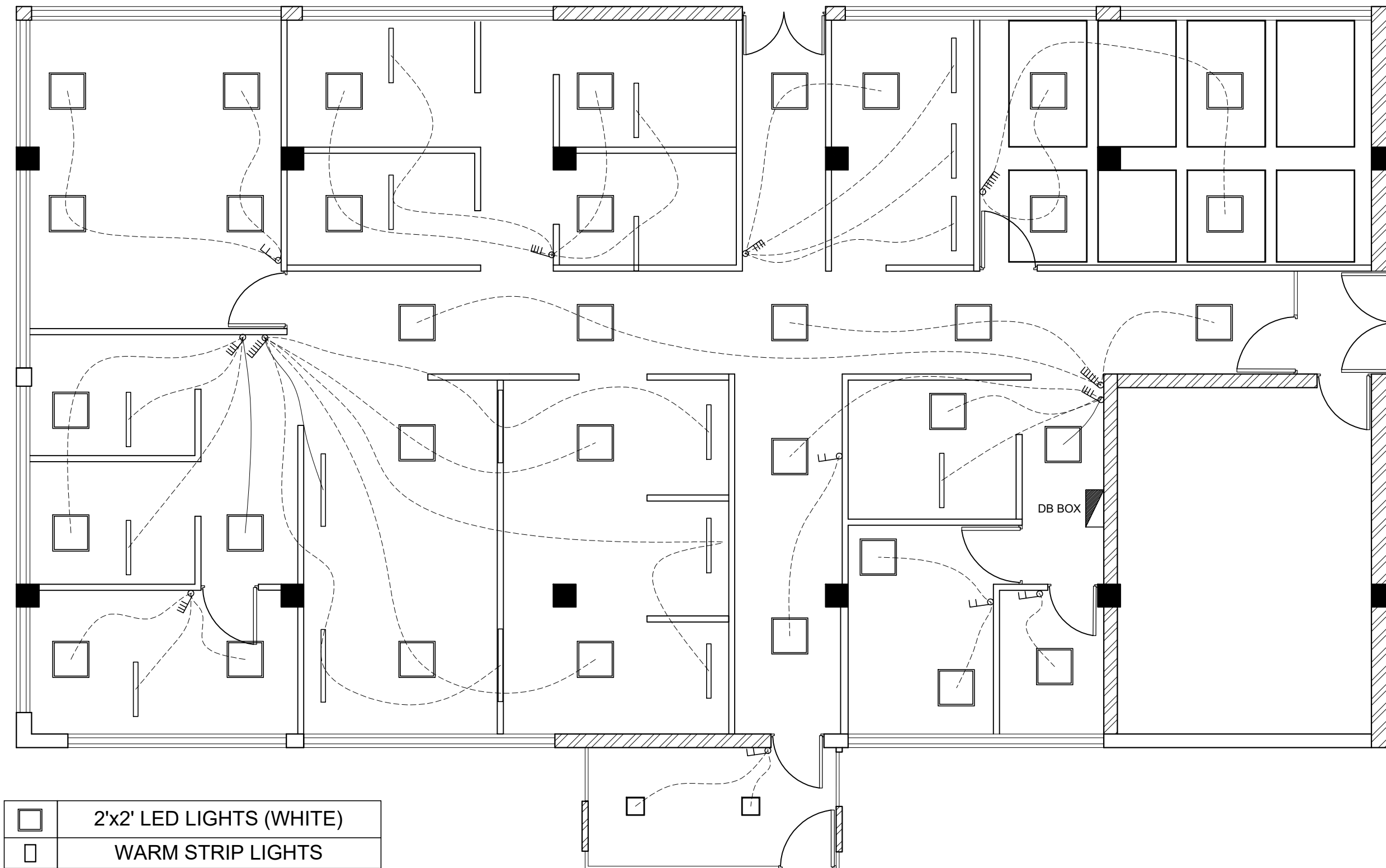
WIRING PLAN SCALE= 1:100
