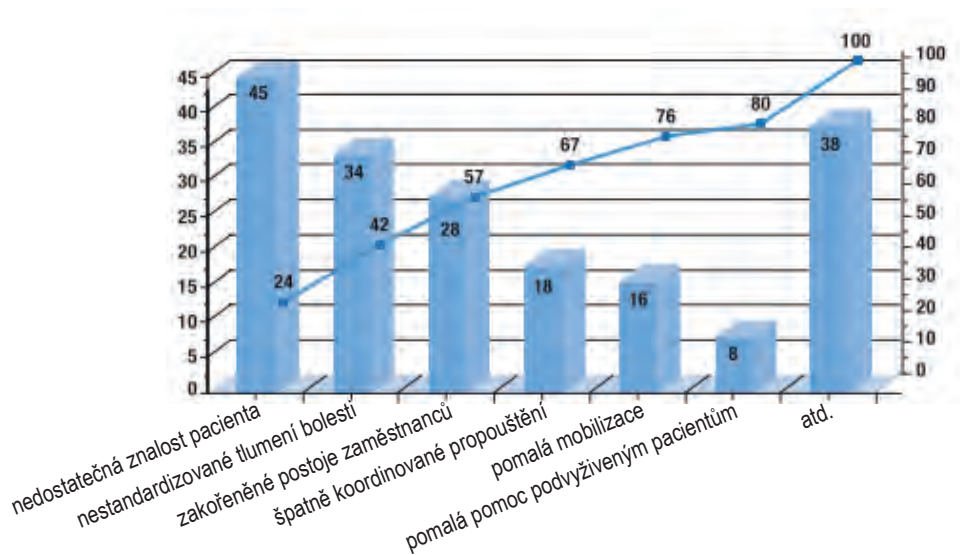
Paretův graf
